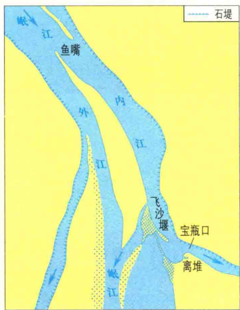
都江堰示意图
